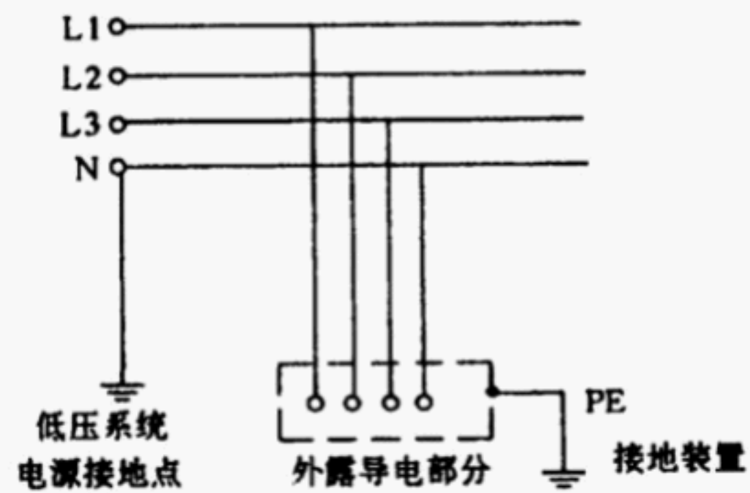
图 4 TT 系统
