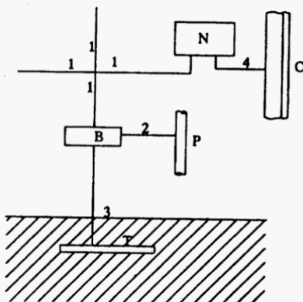
图 6 建筑物内总等电位联结图
