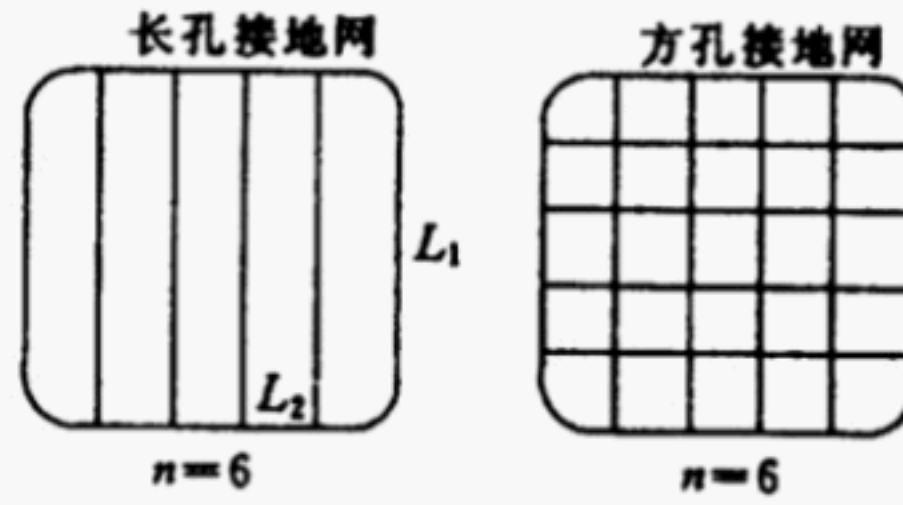
图 B1 接地网的形状
