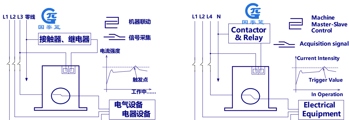
交流常开型 A200K-OA 应用接线参考图
