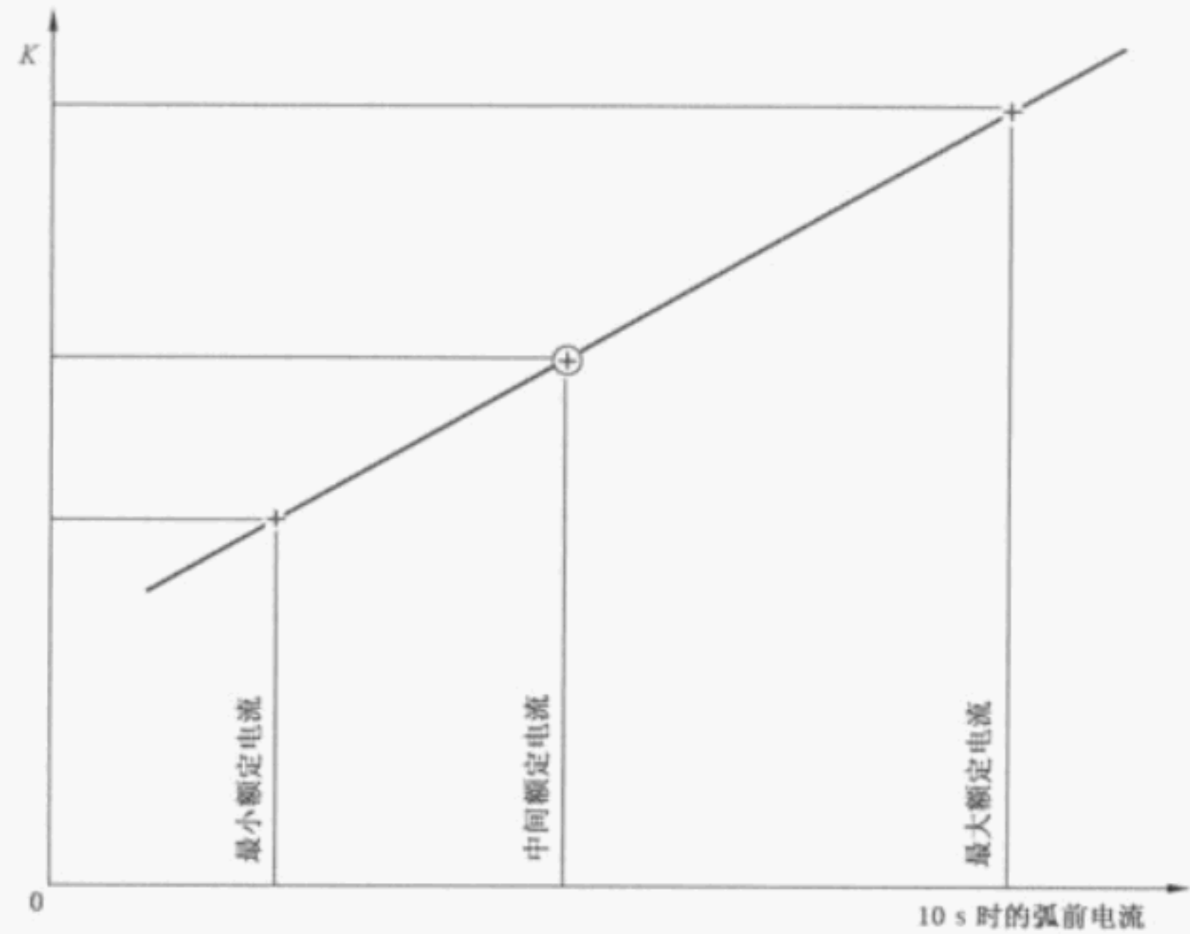
图 1 同族系列中中间额定电流熔断件 K 值的确定
