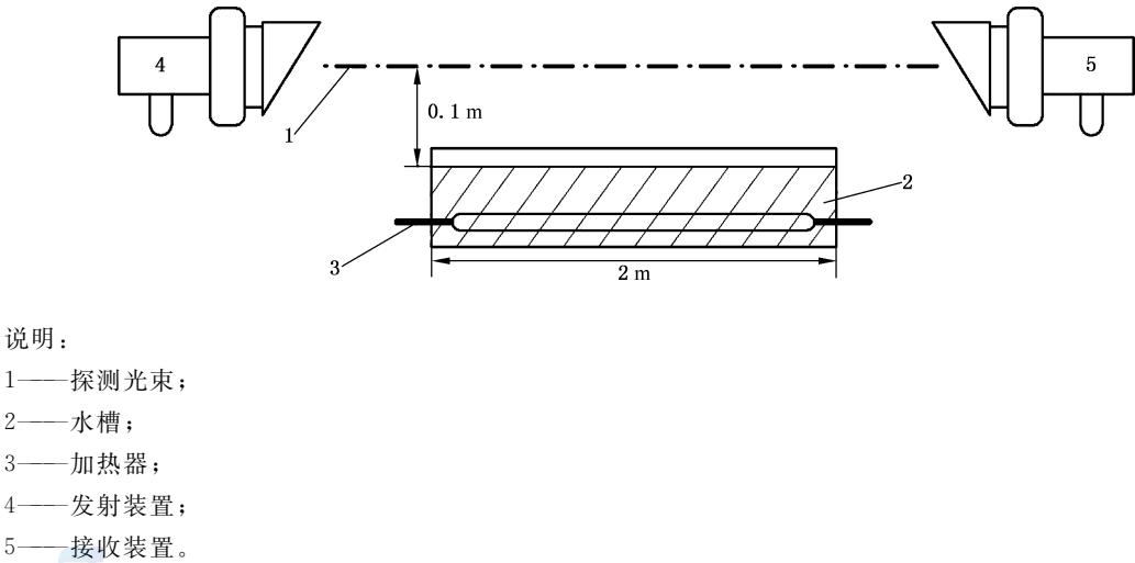
图 A.1 蒸汽干扰试验布置图
